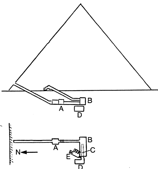
Abb. 18 Mykerinospyramide, Schnitt N-S und Innenanlagen
