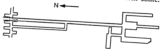
Abb. 7 Unterirdische Anlage (Sarkkammer) der Pyramide des Sechemchet
