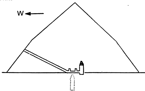
Abb. 12c Schnitt W-O durch die Knickpyramide von Dahschur
