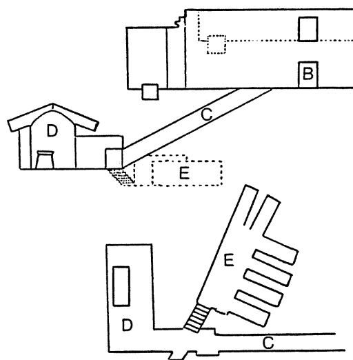
Abb. 19 Mykerinospyramide, Schnitt durch Innenanlagen und Aufsicht auf die hintersten Kammern
