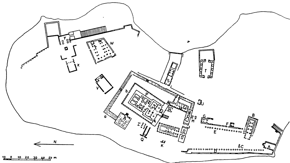
Plan von Philae (Zeichnung von Imtraud Noering, teilweise basierend auf Lyons, teilweise auf Giammarusti-Roccati).
