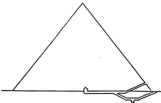
Abb. 17 a Chephrenpyramide bei Gisa, Schnitt N-S
