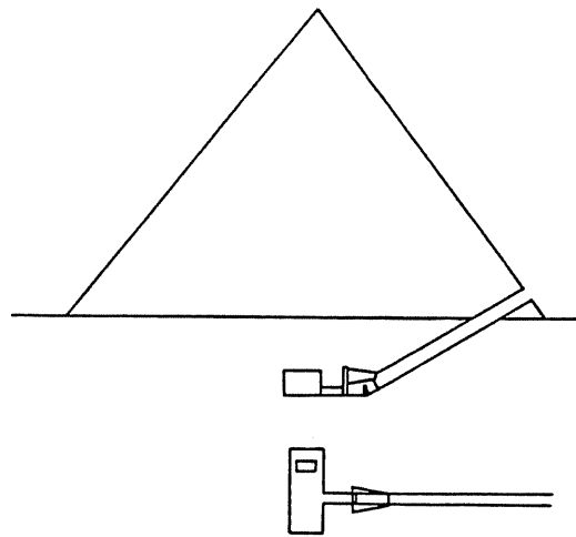
Abb. 20 Kultpyramide des Mykerinos, Schnitt N-S und Aufsicht der Innenanlagen
