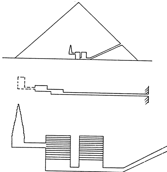
Abb. 14 Rote Pyramide des Snofru von Dahschur, Schnitt N-S, Aufsicht der Innenanlagen und Schnitt durch die Grabkammern
