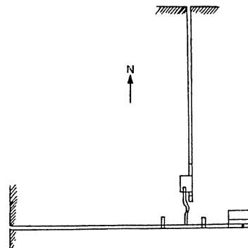
Abb. 12 a Aufsicht auf die Innenanlagen der Knickpyramide von Dahschur
