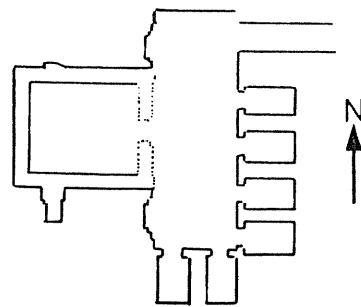
Abb. 22 Innenanlage der Chentkauspyramide
