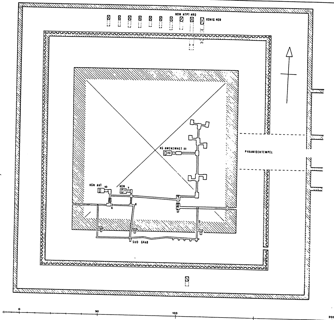
Abb. 27 Pyramide Amenemhets III. bei Dahschur
