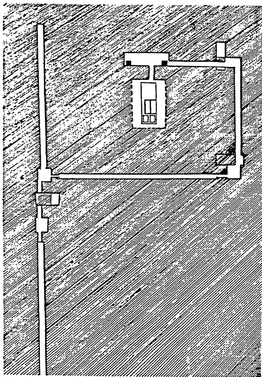
Abb. 28 Innenräume der Pyramide Amenemhats III. in Hawara (nach Fakhry, Pyramids, 223, Abb. 113)
