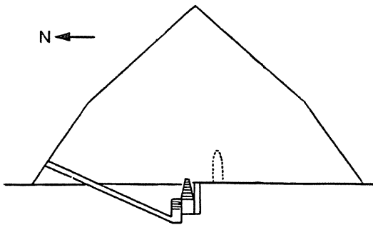
Abb. 12b Schnitt N-S durch die Knickpyramide von Dahschur
