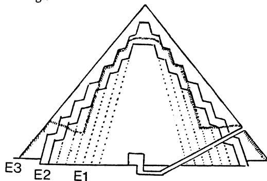
Abb. 11 Schnitt durch die Pyramide von Meidum
