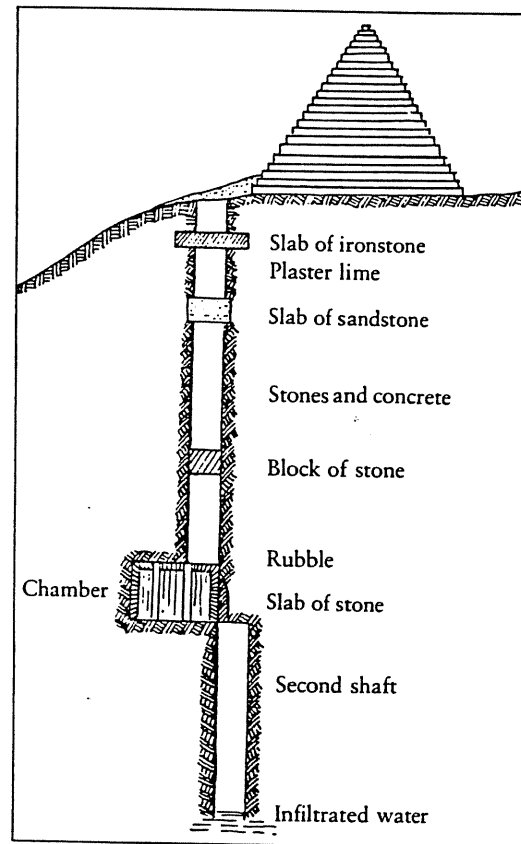
Abb. 29 Schematische Zeichnung einer Pyramidenanlage von Gebel Barkal (nach Ahmed Fakhry, The Pyramids, Chicago 1961, 243 Abb. 121)
